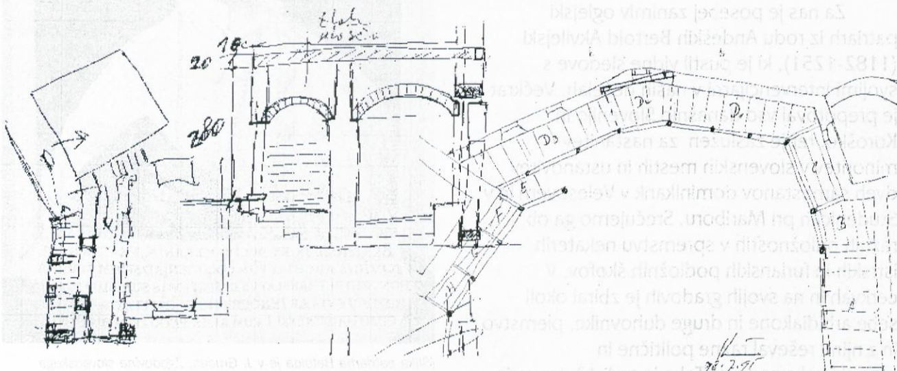
Ing. S. Kerševan: Tehnične študije za obnovo spodnjih arkad na gradu Mirna
